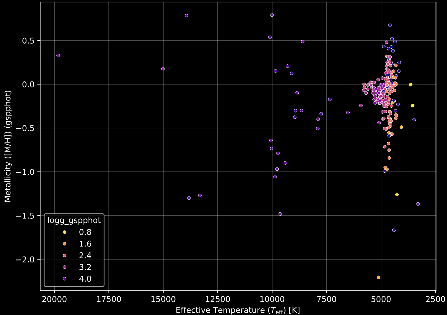
APOGEE DR17 Field: [064+12] Stellar Population Parameters (n= 240)
